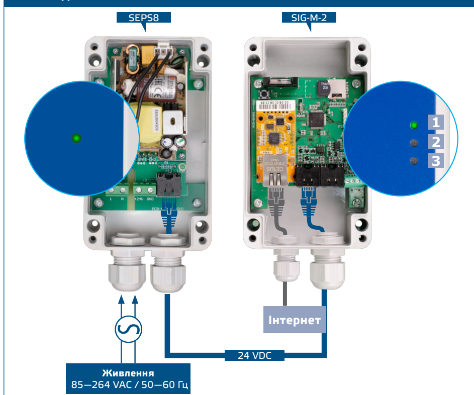
Рис. 6 Підключення кабелю Ethernet LAN
