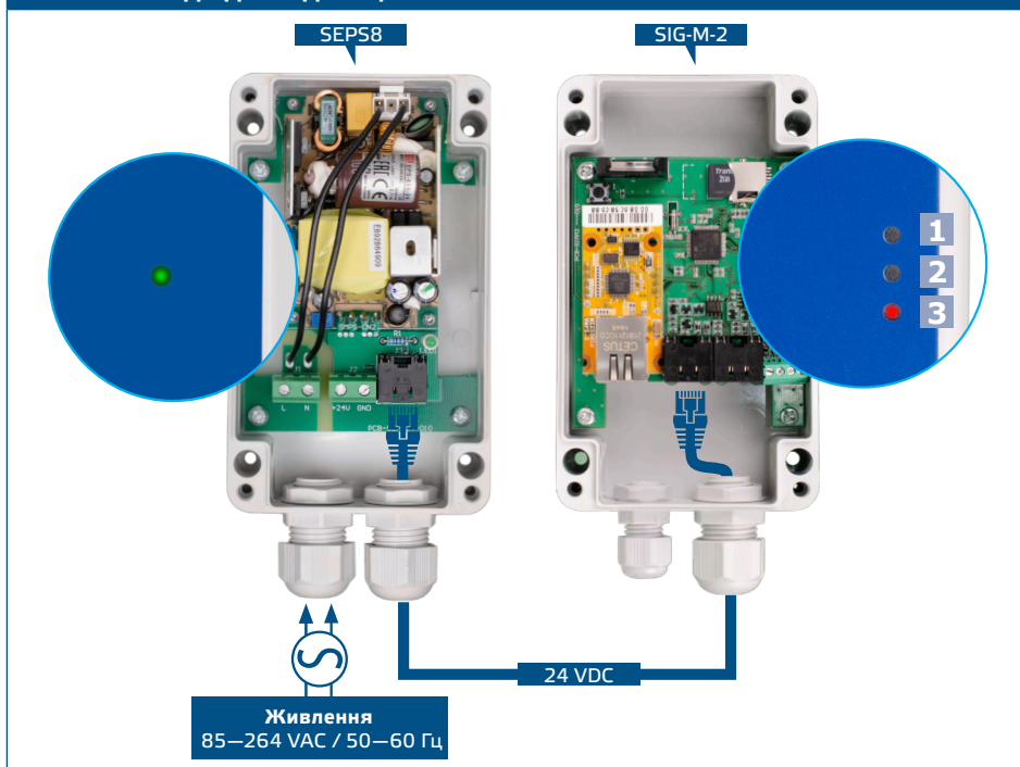
Рис. 5 Світлодіодна індикація
