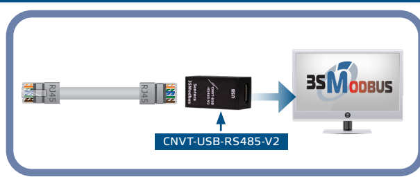
Мал. 5 Підключення 3SModbus RJ45
