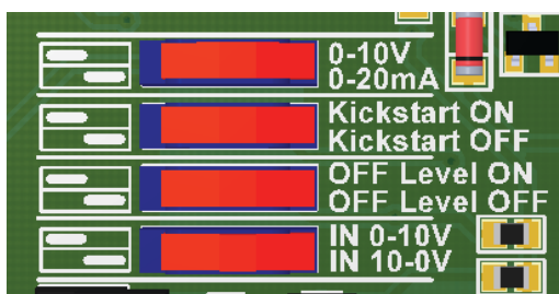
Мал. 4 налаштування DIP-перемикача
