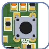
Мал. 10 Калібрування датчика і тактовий перемикач скидання реєстра Modbus
