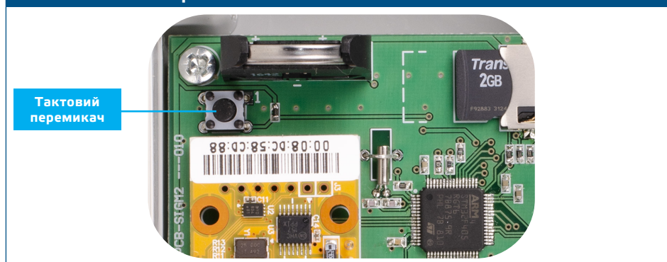
Мал. 4 Тактовий перемикач
