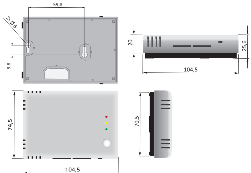
Мал. 2 Монтажні розміри
