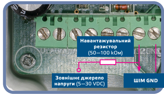
Мал. 6 Приклад підключення ШІМ (з відкритим колектором)
