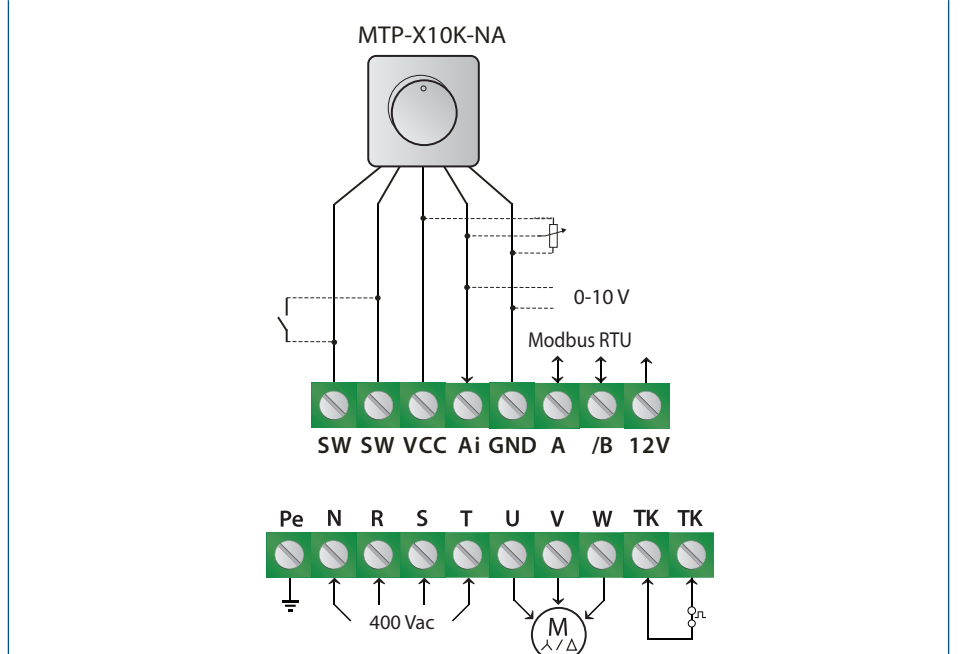
Şek. 3 Kablolama ve bağlantılar
