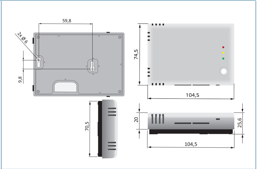
Şek. 2 Montaj boyutu
