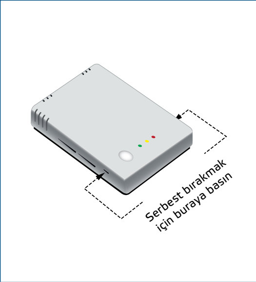
Şek. 1 Geçmelerin serbest bırakılması
