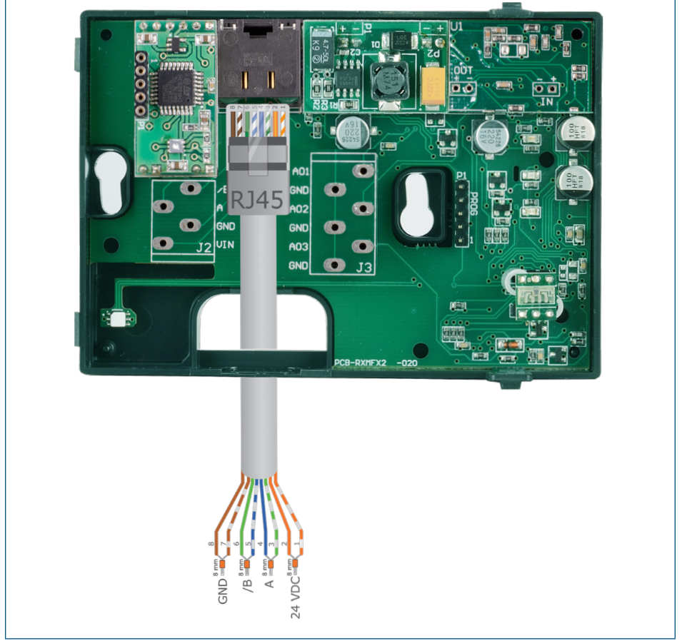
Şek. 4 Kablolama
