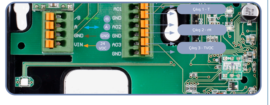
Şek. 4 Kablolama
