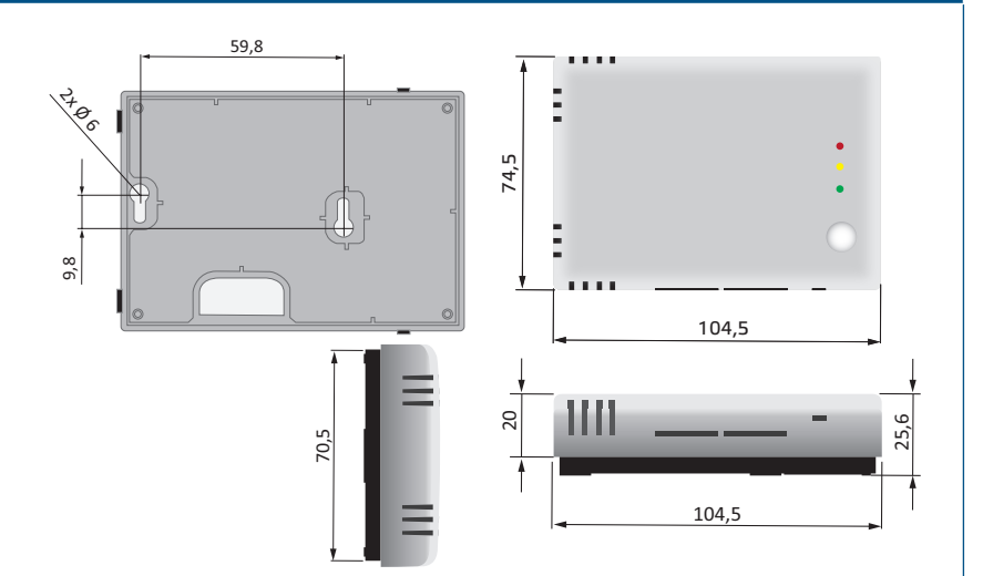
Şek. 2 Montaj boyutları
