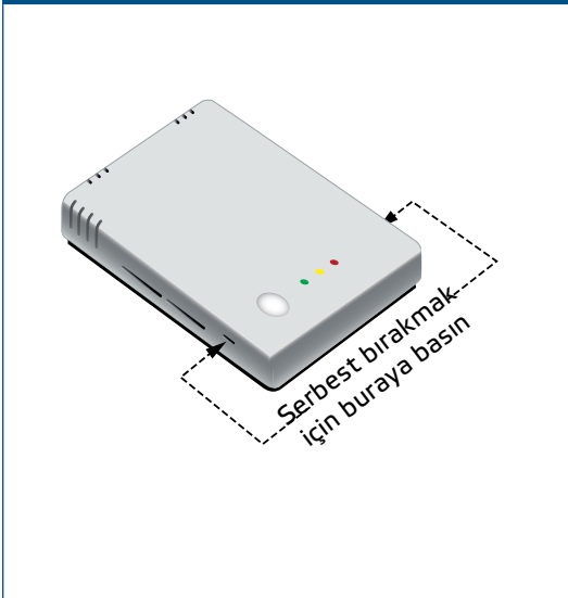
Şek. 1 Geçmeli bağlantıları serbest bırakma
