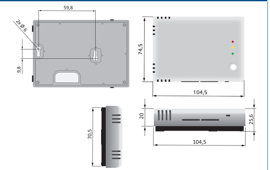
Şek. 2 Montaj boyutları
