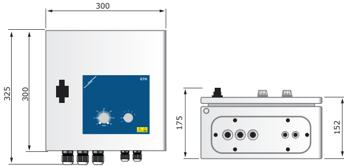
Fig. 1 Montaj boyutları
