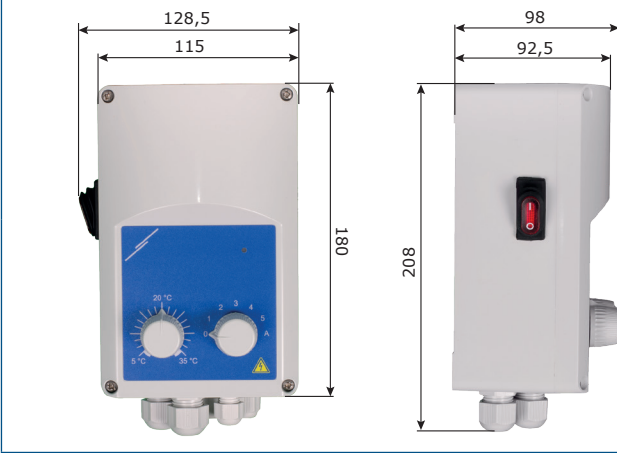
Şek. 1 Montaj boyutları
