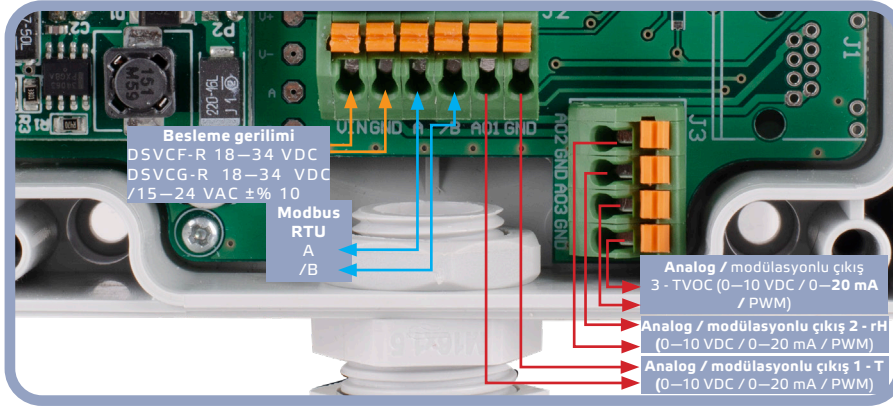
Şek. 4 Kablolama ve bağlantılar
