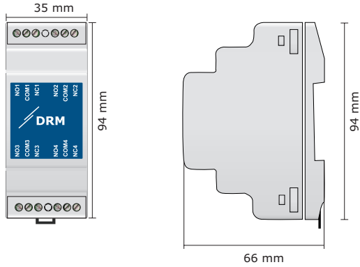
Şek. 1 Montaj boyutları
