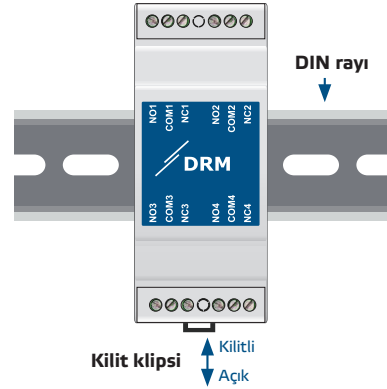
Şek. 2 Montaj konumu
