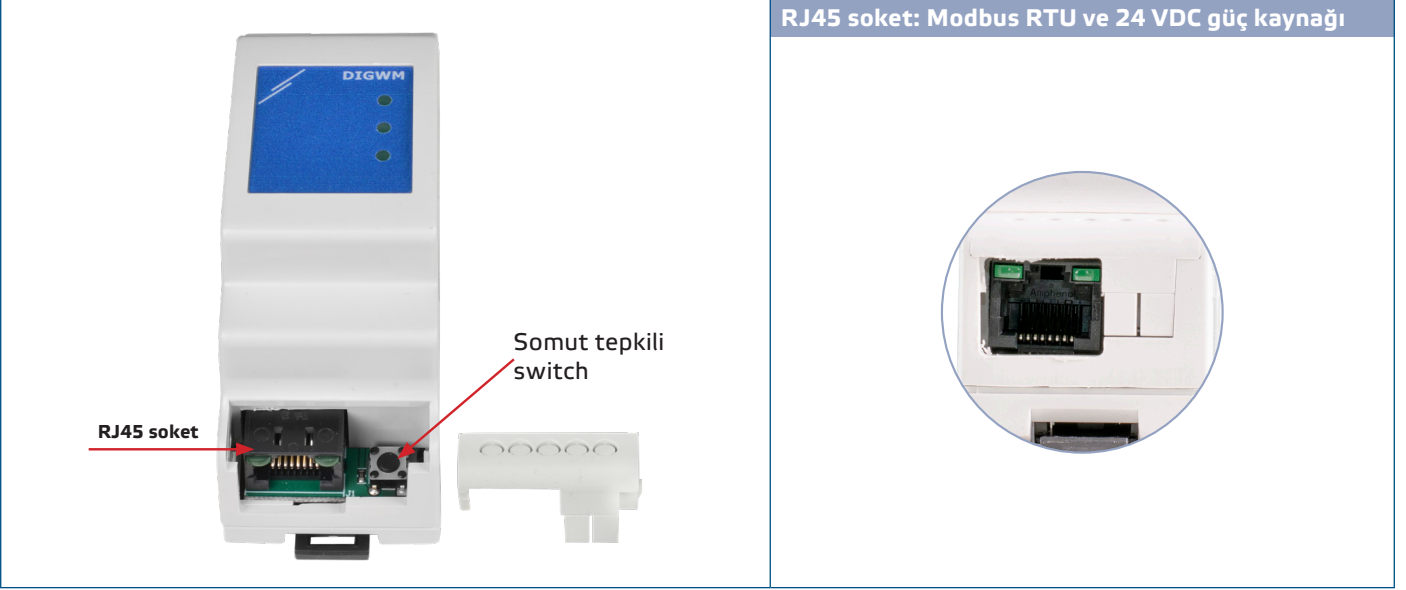
Şek. 3 Kabloleme ve bağlantılar
