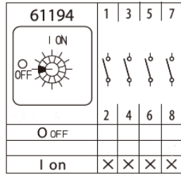
Anahtarlama diyagramı 61194
