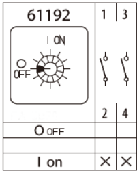
Anahtarlama diyagramı 61192
