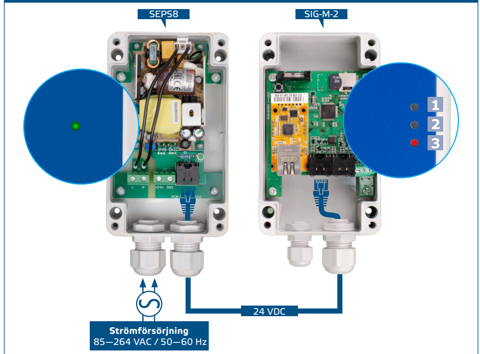
Fig. 5 LED-indikeringar
