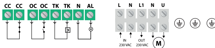
Fig. 3 Koppling och anslutningar
