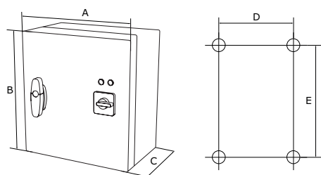
Fig. 1 Monteringsmått
