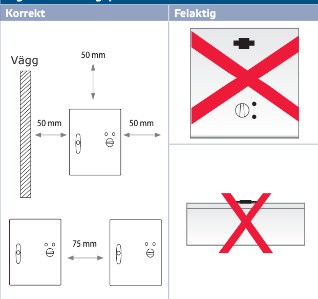
Fig. 2 Monteringsposition
