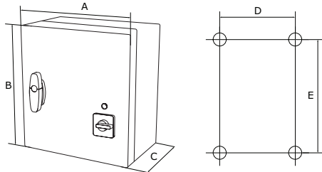
Bild 1 Monteringsmått
