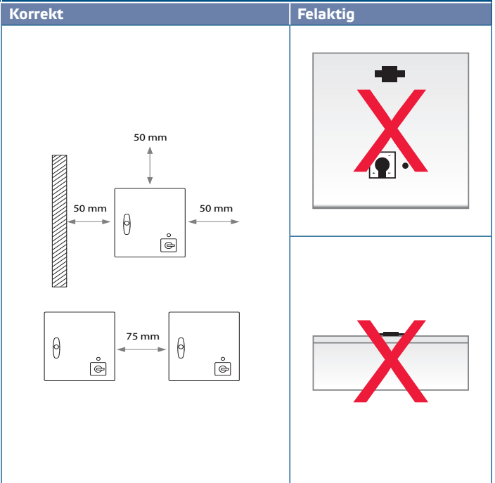
Bild 2 Monteringsposition
