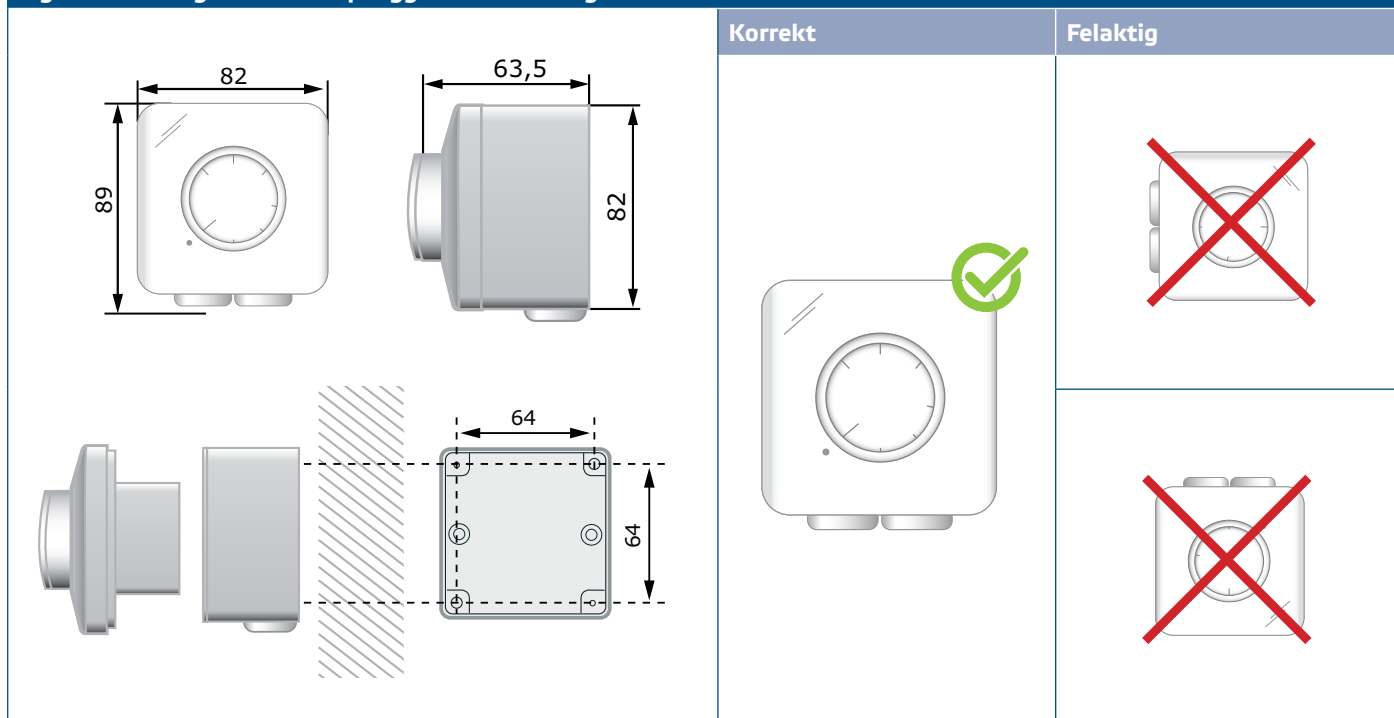
Fig. 3 Monteringsmått - utanpåliggande montering
