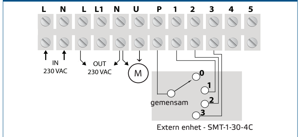
Fig. 3 Kopplingsdiagram
