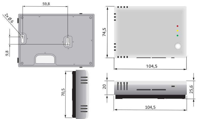
Fig. 2 Monteringsmått
