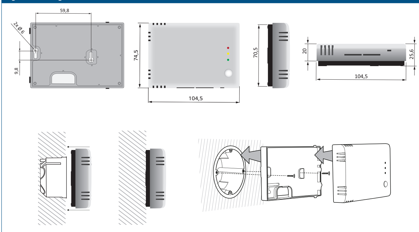
Fig. 2 Monteringsmått
