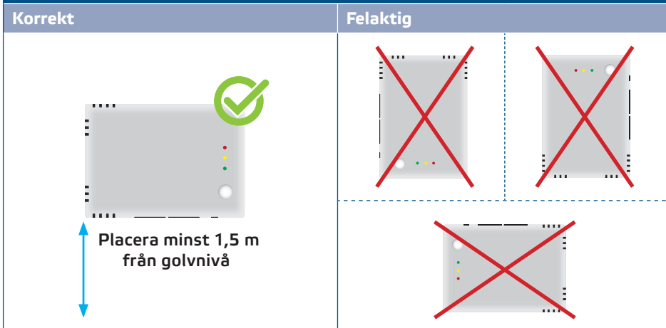
Fig. 3 Monteringsposition
