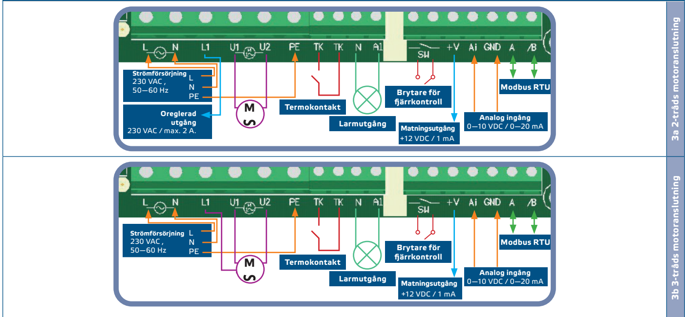
Fig. 3 Kopplingschema
