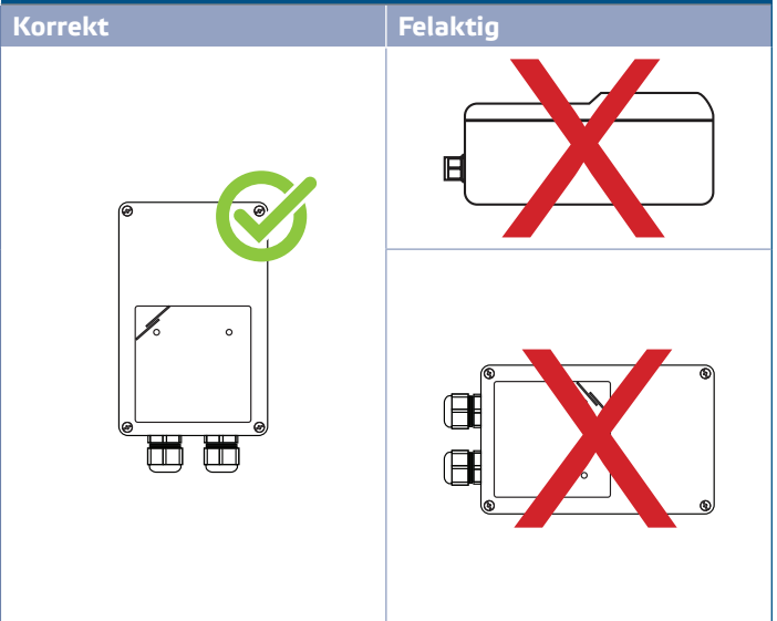
Fig. 2 Monteringsposition
