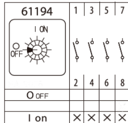
Växlingsdiagram 61194
