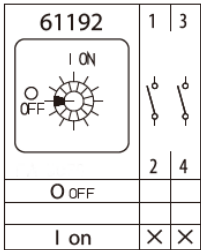
Växlingsdiagram 61192
