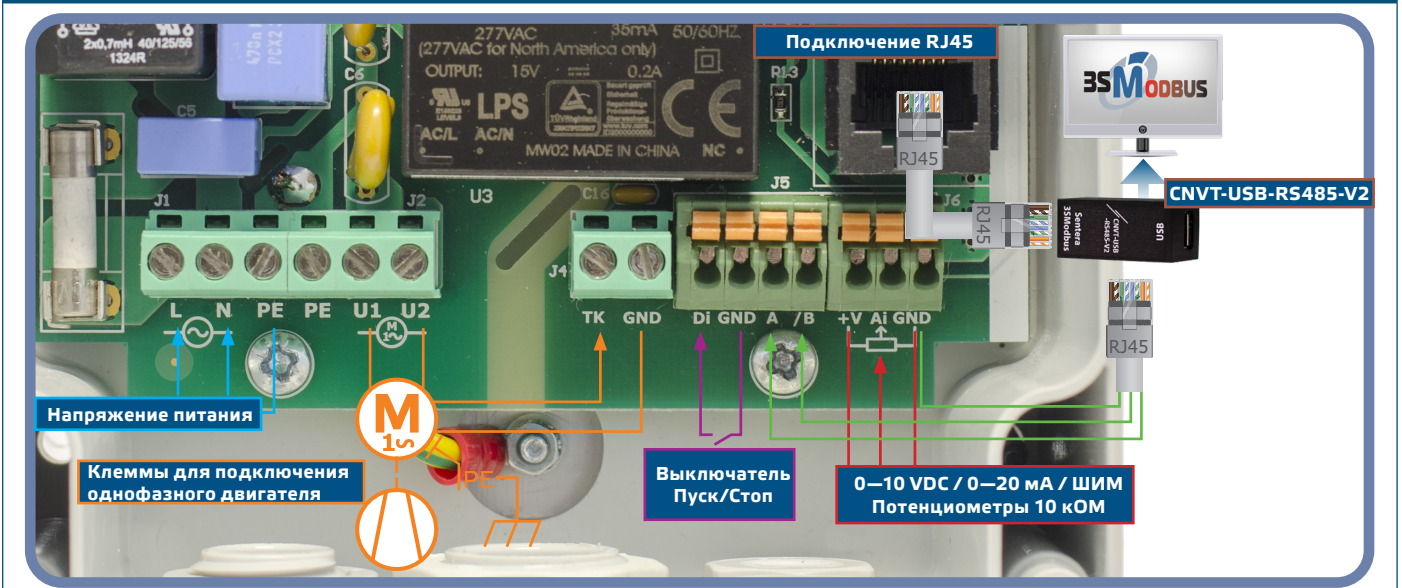
Рис. 1 Схема соединения
