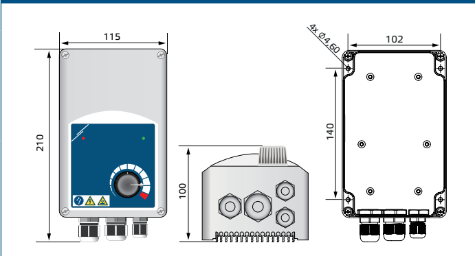
Рис. 2 Монтажные размеры
