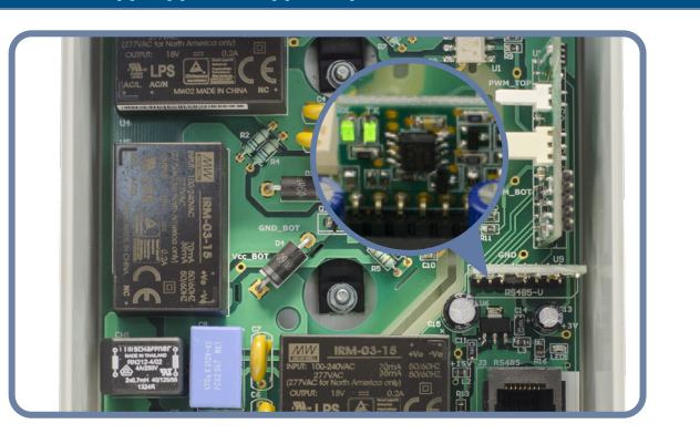
Рис. 8 Светодиодная индикация связи
