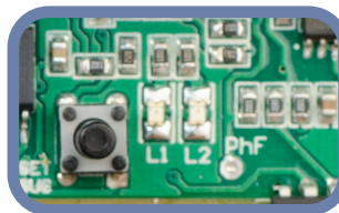
Рис. 10 Индикация обнаружения связи
