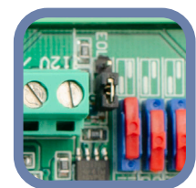
Рис. 8 Перемычка резистора сетевой шины
