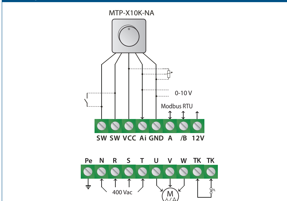
Рис. 3 Проводка и соединения
