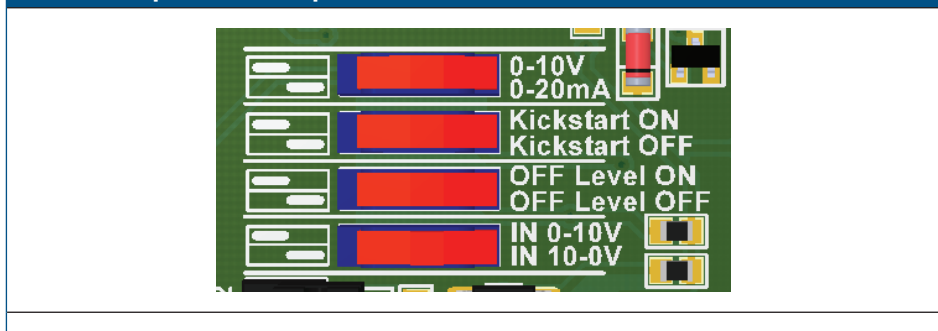
Рис. 4 Настройки DIP-переключателя
