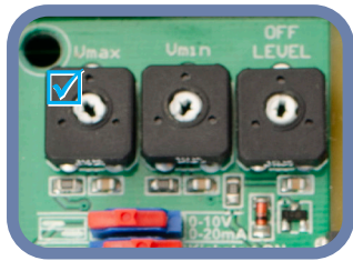
Рис. 5 Максимальная скорость подстроечного резистора
