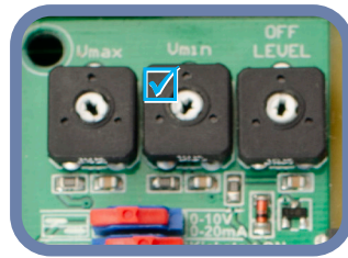
Рис. 6 Минимальная скорость подстроечного резистора
