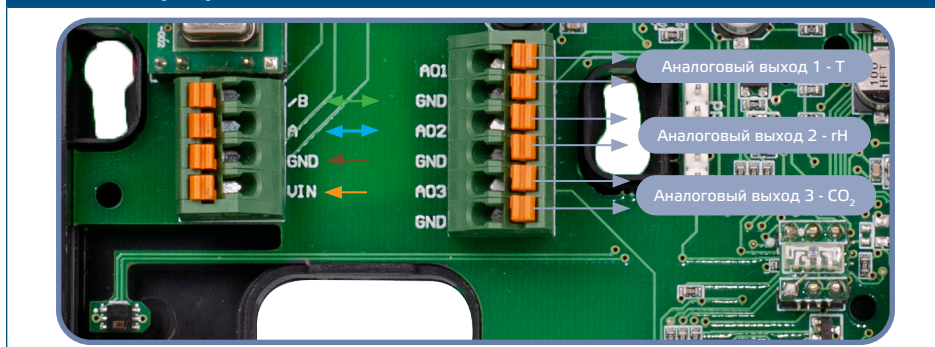
Рис.4 Электропроводка
