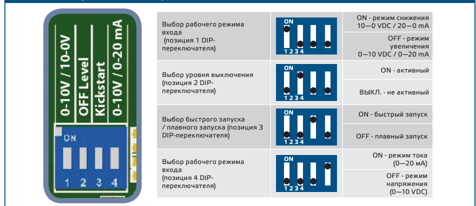
Рис. 4 Настройки DIP-переключателя
