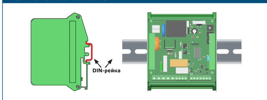
Рис. 2 Монтажное положение
