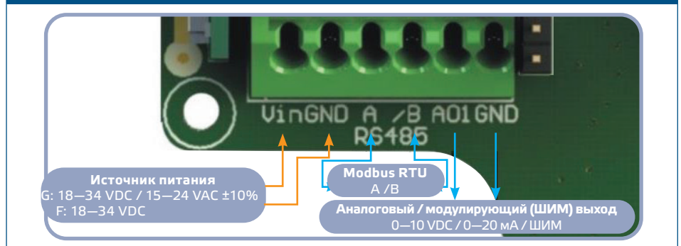
Рис.3 Соединения
