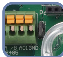
Рис. 5 Переключатель подтягивающего резистора 1
