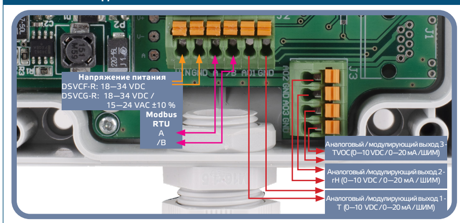
Рис. 4 Схема подключения
