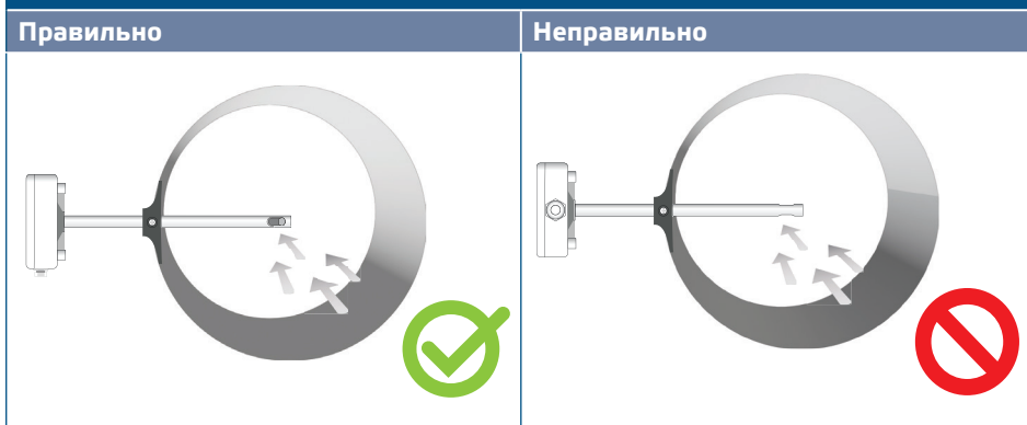
Рис. 2 Монтажное положение
