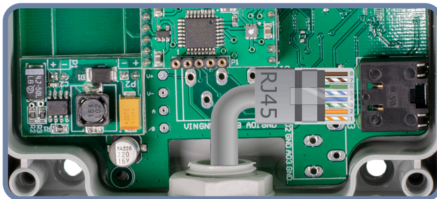
Рис. 4 Схема подключения
