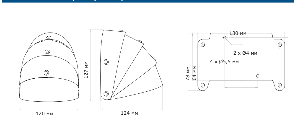
Рис. 2 Монтажные размеры - встроенный монтаж
