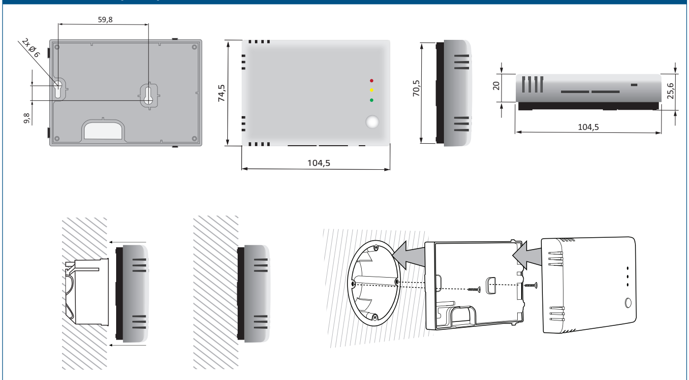
Рис. 2 Монтажные размеры
