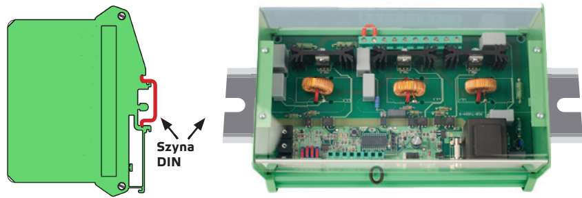
Rys. 2 Pozycja montażowa
