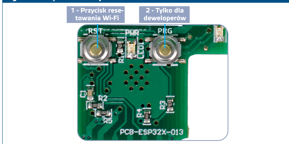
Figa. 5 Przełącznik taktacji resetowania Wi-Fi
