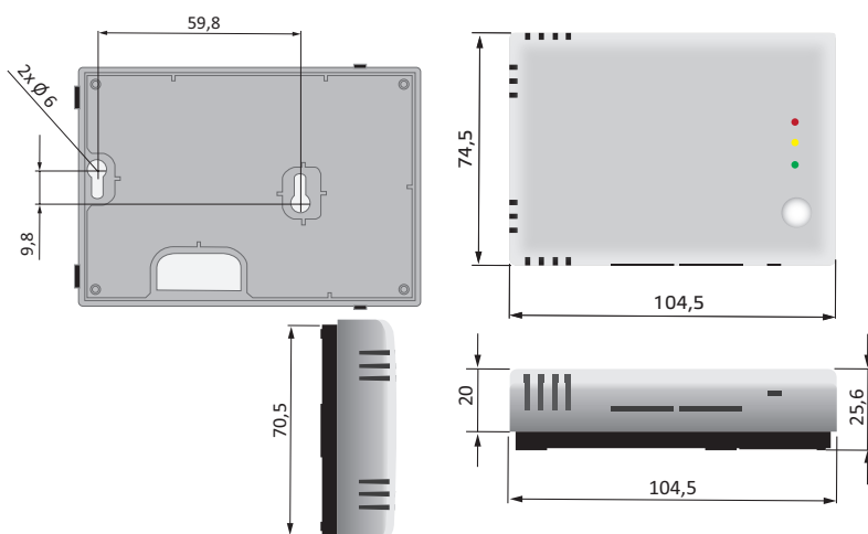
Rys. 2 Wymiary montażowe
