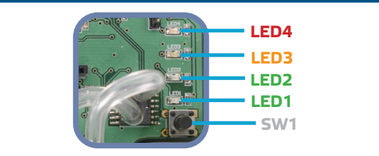
Rys. 8 Kalibracja czujnika i reset rejestrów Modbus
