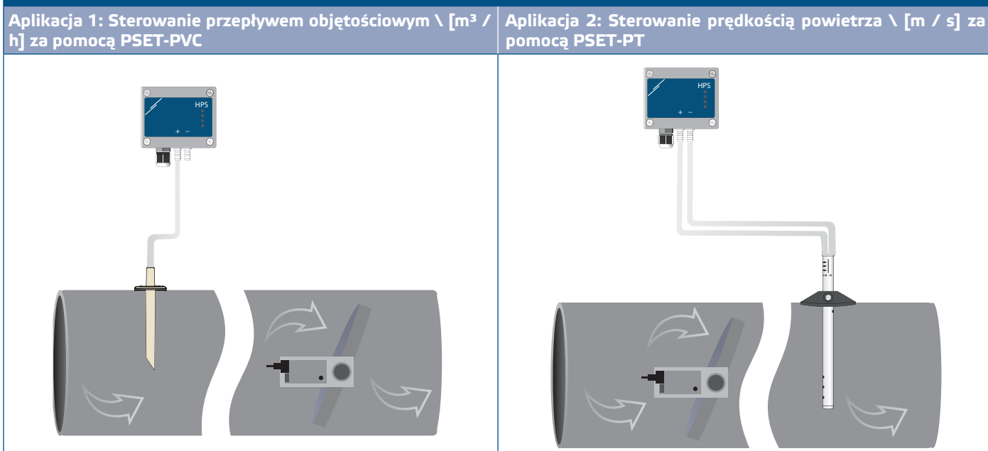
Rys. 4 Podłączenie z akcesoriami
