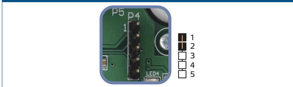
Rys. 10 Zworka resetująca rejestr przytrzymujący Modbus
