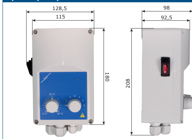
Rys. 1 Wymiary montażowe
