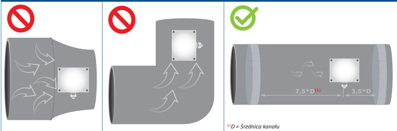
Rys. 3 Wymagania montażowe
