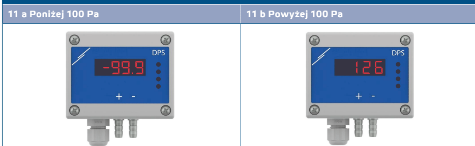
Rys. 11 Wskaźnik różnicy ciśnień
