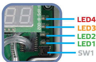
Rys. 8 Kalibracja czujnika i reset rejestru Modbus
