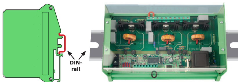
Fig. 2 Montagepositie
