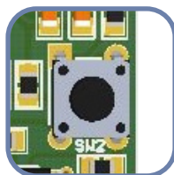
Fig. 10 Sensorkalibratie en drukknop voor Modbus-registerreset
