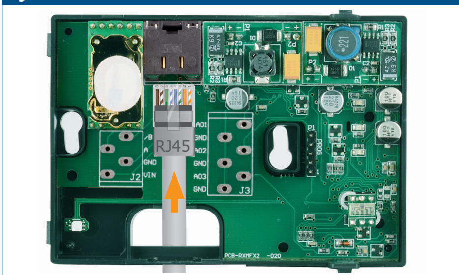
Fig. 4 Aansluitschema
