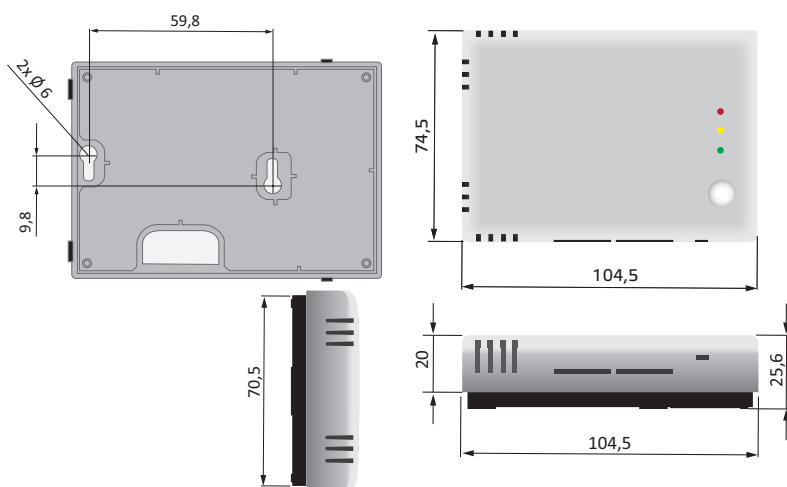
Fig. 2 Afmetingen
